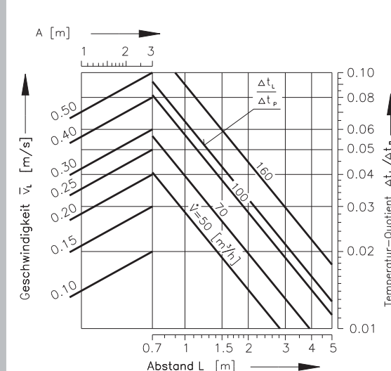
Diagramm 2 Luftgeschwindigkeit und Temperaturdifferenz
