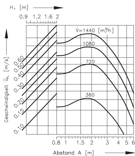
Diagramm 24 Mehrreihige Anordnung der Dralldurchlässe, wenn B = 3 m
