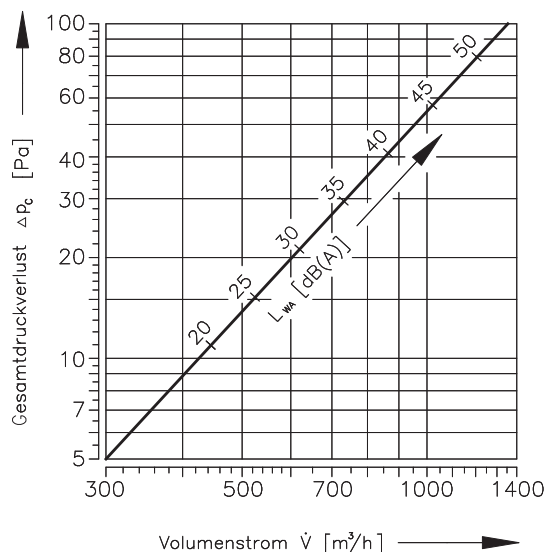
Diagramm 17 Druckverlust und Schalleistung
