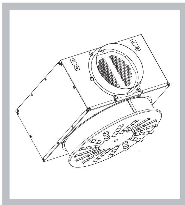
Abb. 2 VVM mit Anschlusskasten - Runde Frontplatte
