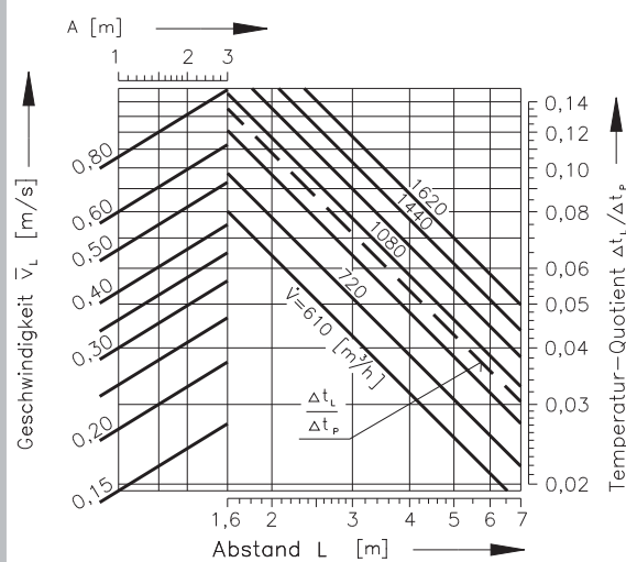
Diagramm 26 Luftgeschwindigkeit und Temperaturdifferenz
