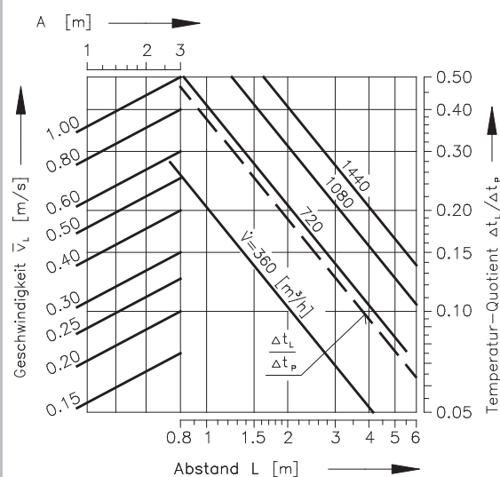
Diagramm 22 Luftgeschwindigkeit und Temperaturdifferenz
