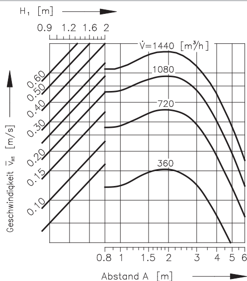
Diagramm 19 Einreihige oder mehrreihige Anordnung der Dralldurchlässe, wenn B \geq 4 m
