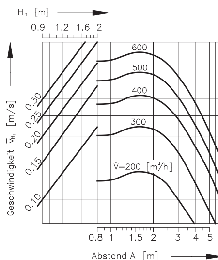
Diagramm 16 Mehrreihige Anordnung der Dralldurchlässe, wenn B = 3 m
