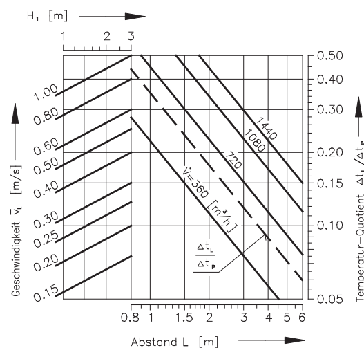
Diagramm 18 Luftgeschwindigkeit und Temperaturdifferenz
