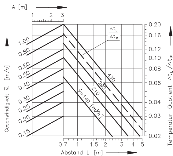
Diagramm 10 Luftgeschwindigkeit und Temperaturdifferenz
