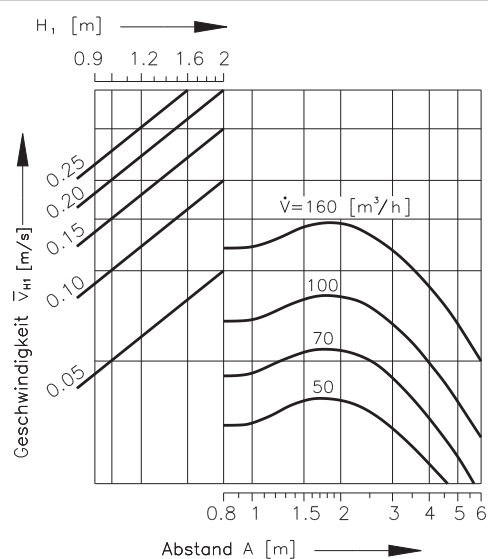
Diagramm 3 Einreihige oder mehrreihige Anordnung der Dralldurchlässe, wenn B \geq 4 m
