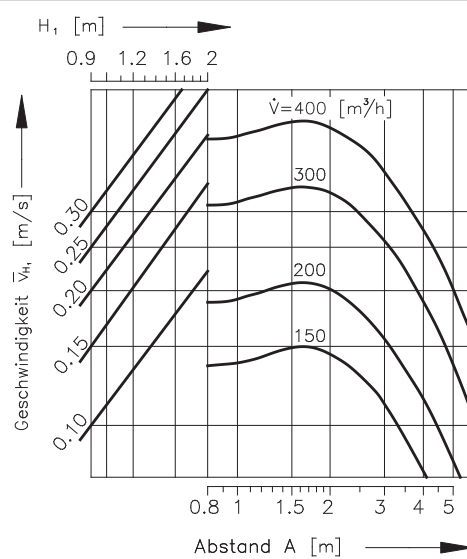
Diagramm 8 Mehrreihige Anordnung der Dralldurchlässe, wenn B = 3 m
