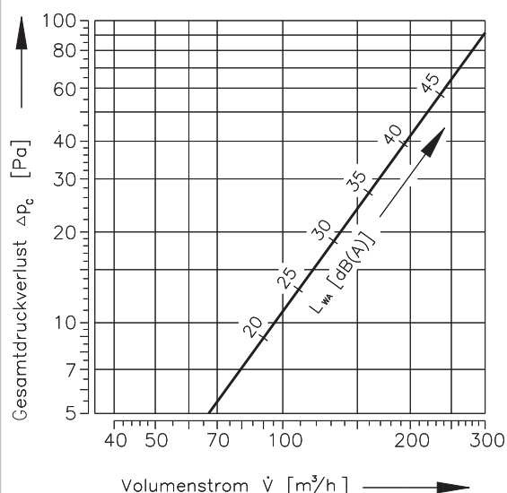
Diagramm 3 Einreihige oder mehrreihige Anordnung der Dralldurchlässe, wenn B \geq 4 m
