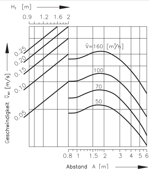
Diagramm 4 Mehrreihige Anordnung der Dralldurchlässe, wenn B = 3 m
