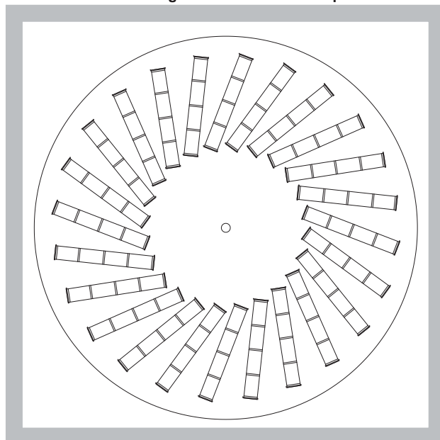
Abb. 4 Ausführung VVM/K - Runde Frontplatte
