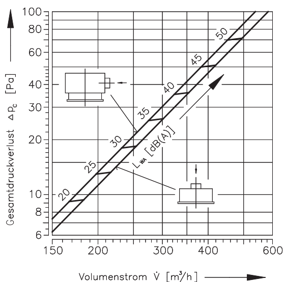
Diagramm 5 Druckverlust und Schalleistung
