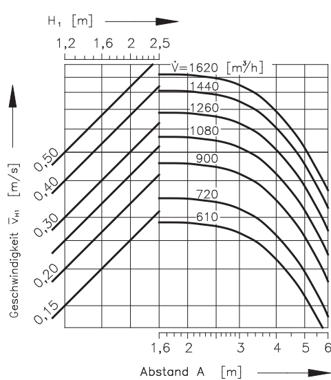
Diagramm 28 Mehrreihige Anordnung der Dralldurchlässe, wenn B = 3 m
