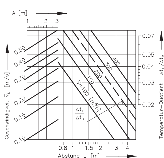
Diagramm 6 Luftgeschwindigkeit und Temperaturdifferenz
