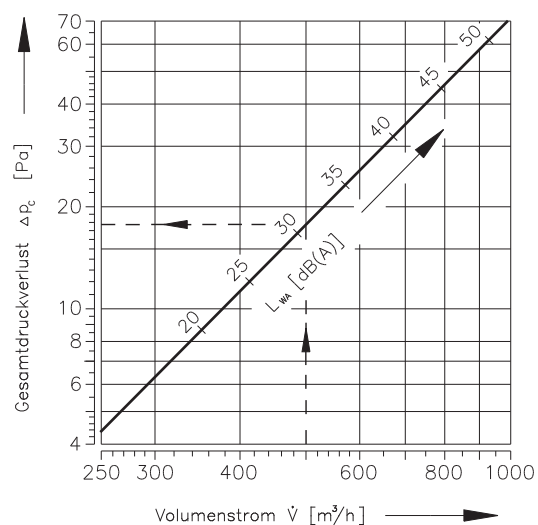
Diagramm 13 Druckverlust und Schalleistung
