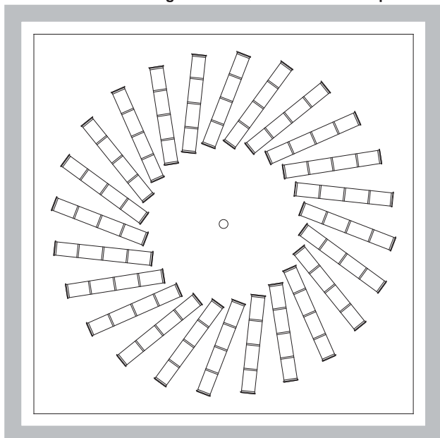
Abb. 3 Ausführung VVM/C - Quadratische Frontplatte
