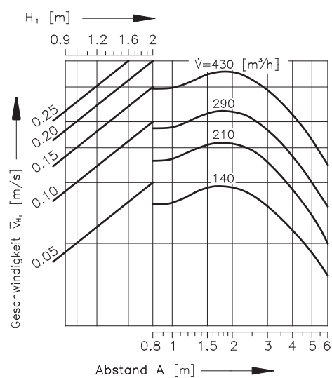
Diagramm 12 Mehrreihige Anordnung der Dralldurchlässe, wenn B = 3 m
