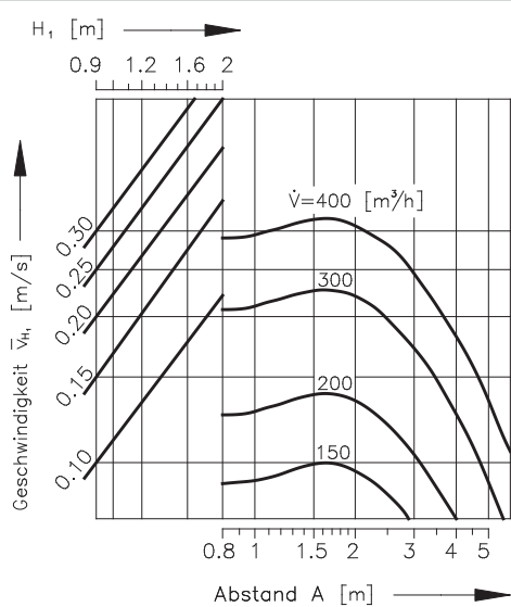
Diagramm 7 Einreihige oder mehrreihige Anordnung der Dralldurchlässe, wenn B \geq 4 m
