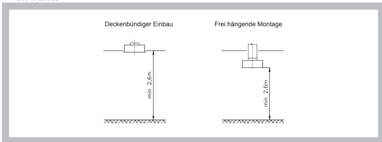
Abb. 11 Befestigungsart
