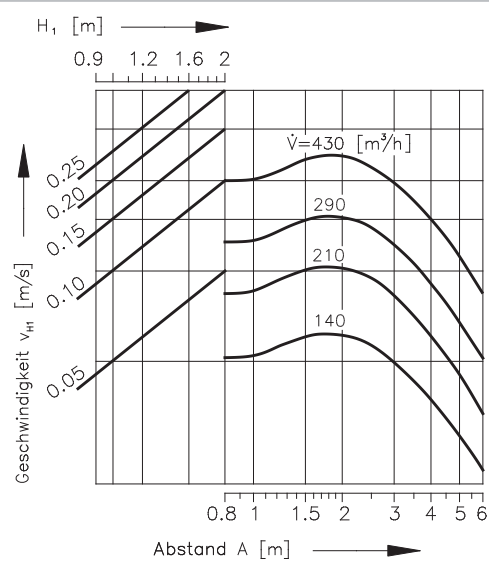
Diagramm 11 Einreihige oder mehrreihige Anordnung der Dralldurchlässe, wenn B \geq 4 m
