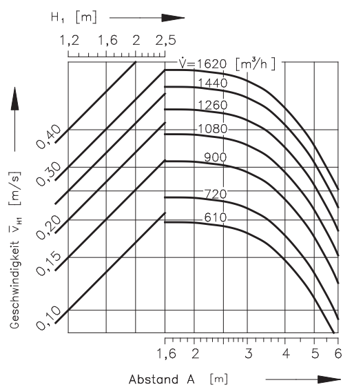
Diagramm 27 Einreihige oder mehrreihige Anordnung der Dralldurchlässe, wenn B \geq 4 m
