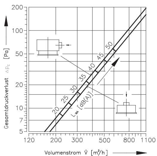
Diagramm 9 Druckverlust und Schalleistung
