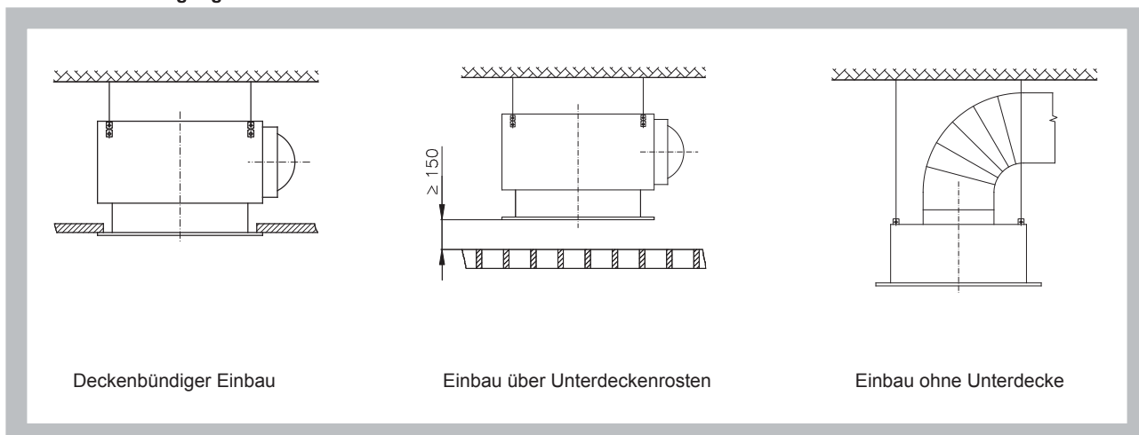
Abb. 11 Befestigungsart
