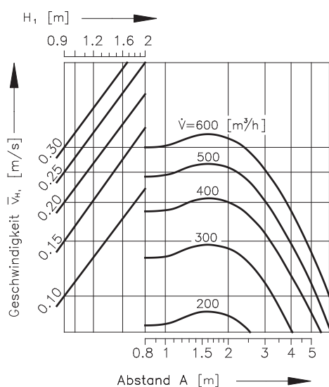
Diagramm 15 Einreihige oder mehrreihige Anordnung der Dralldurchlässe, wenn B \geq 4 m
