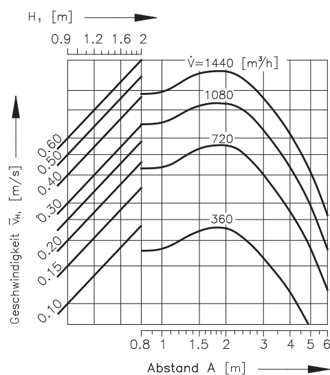
Diagramm 20 Mehrreihige Anordnung der Dralldurchlässe, wenn B = 3 m
