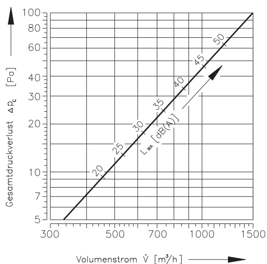
Diagramm 21 Druckverlust und Schalleistung
