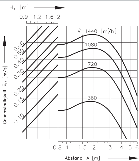
Diagramm 23 Einreihige oder mehrreihige Anordnung der Dralldurchlässe, wenn B \geq 4 m
