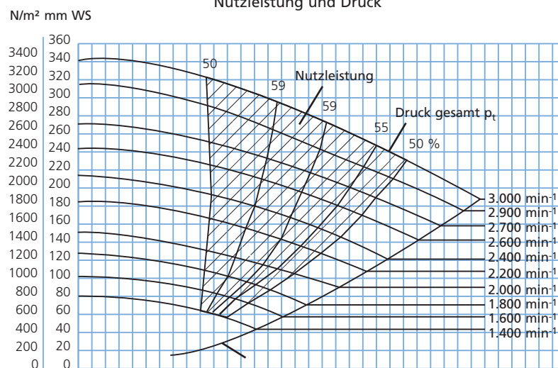
Nutzleistung und Druck
